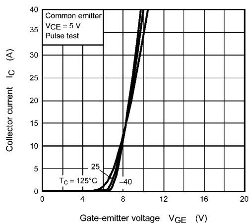
Fig. 8.5 I_C - V_{GE}
