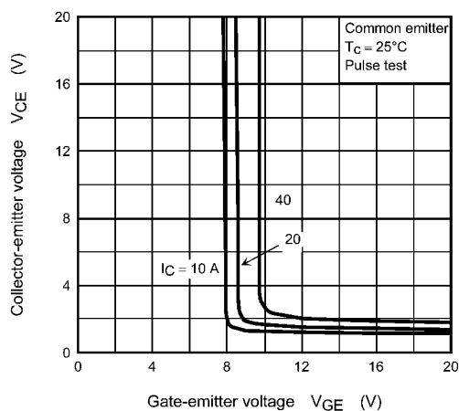
Fig. 8.3 V_{CE} - V_{GE}
