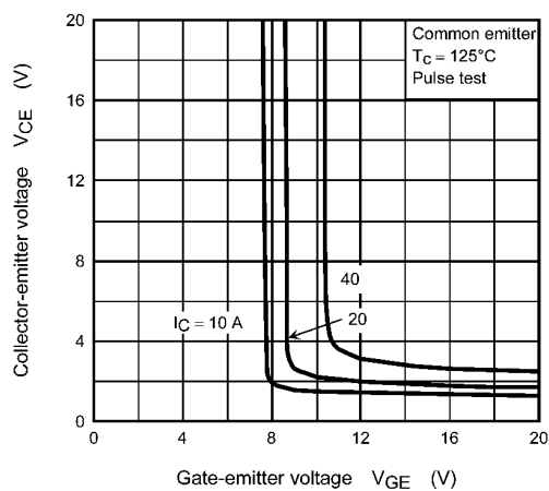
Fig. 8.4 V_{CE} - V_{GE}
