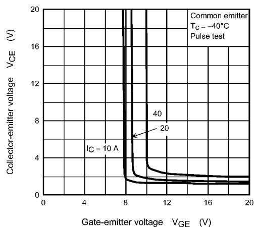
Fig. 8.2 V_{CE} - V_{GE}
