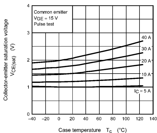
Fig. 8.6 V_{CE(sat)} - T_c
