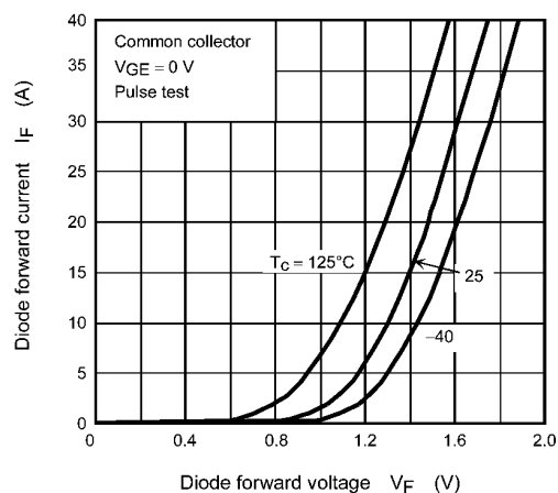
Fig. 8.14 I_F - V_F
