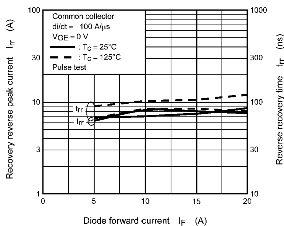
Fig. 8.15 I_{RR} , t_r - I_F
