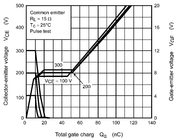
Fig. 8.13 V_{CE} , V_{GE} - Q_g
