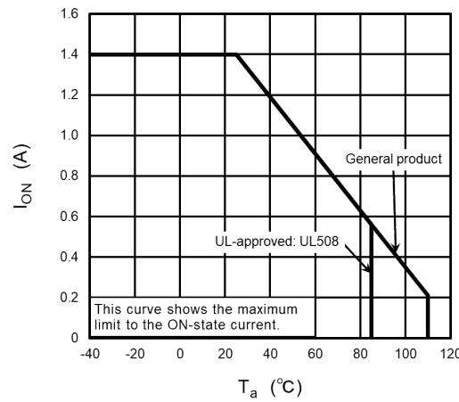
Fig. 14.1.2 I_{ON} - T_a
