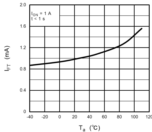
Fig. 14.1.6 I_{FT} - T_a
