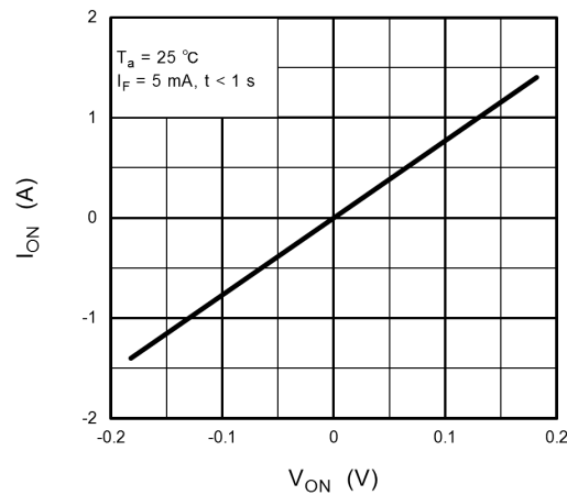
Fig. 14.1.4 I_{ON} - V_{ON}
