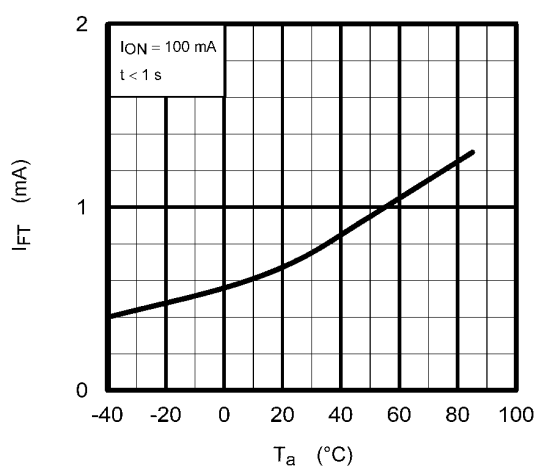
Fig. 12.1.6 I_{FT} - T_a
