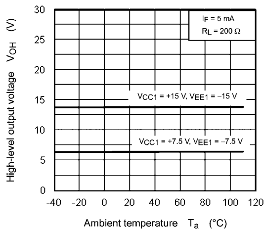
Fig. 13.2.8 V_{OH} - T_a
